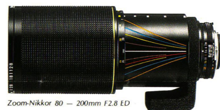
Zoom-Nikkor 80-200mm F2.8 ED
